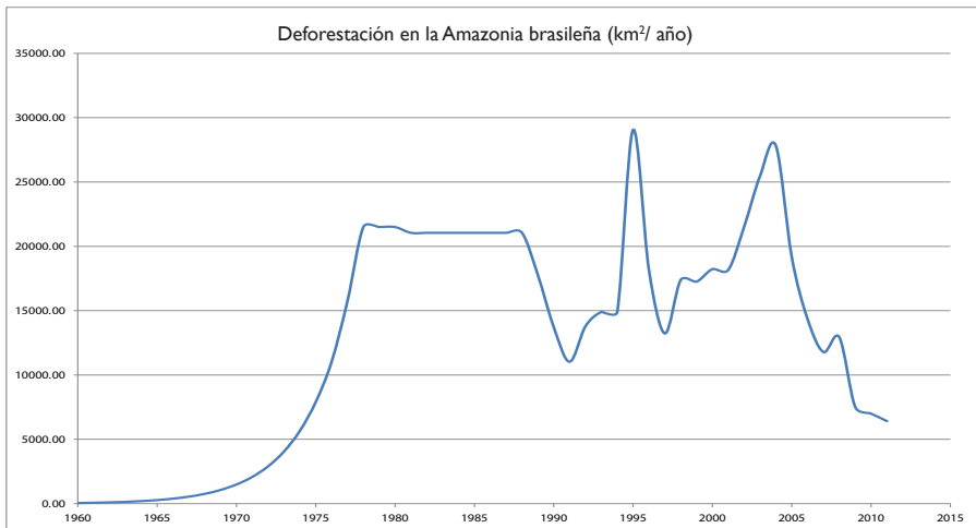
Gráfico 3. Deforestación en la Amazonia brasileña: 1960-2011
