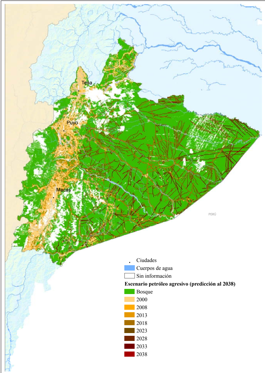
Mapa 5. Escenario petrolero agresivo (predicción al 2038)
